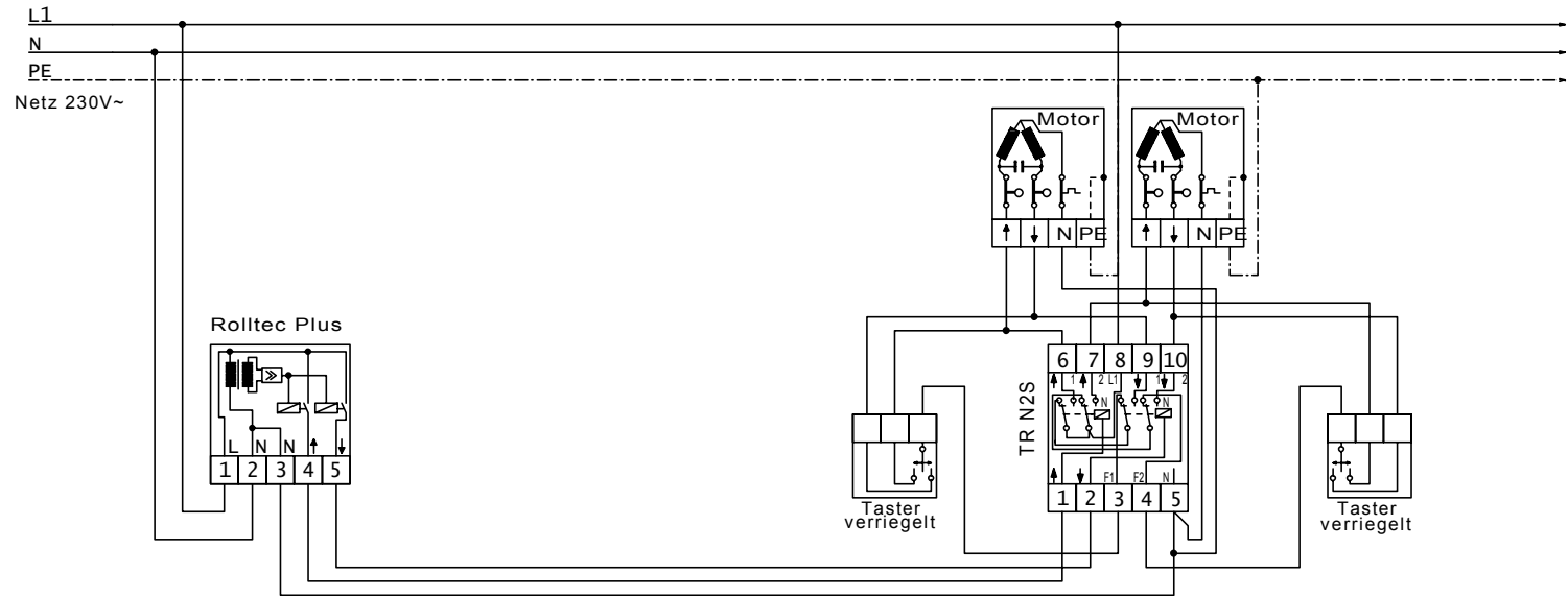
Die Klemmenbelegung der Rolltec Plus entspricht der Klemmenbelegung des VestaLogo
